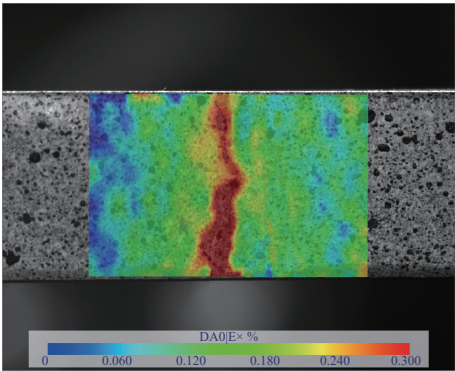
图 5 焊趾处应变场 Fig. 5 Strain field at weld toe
