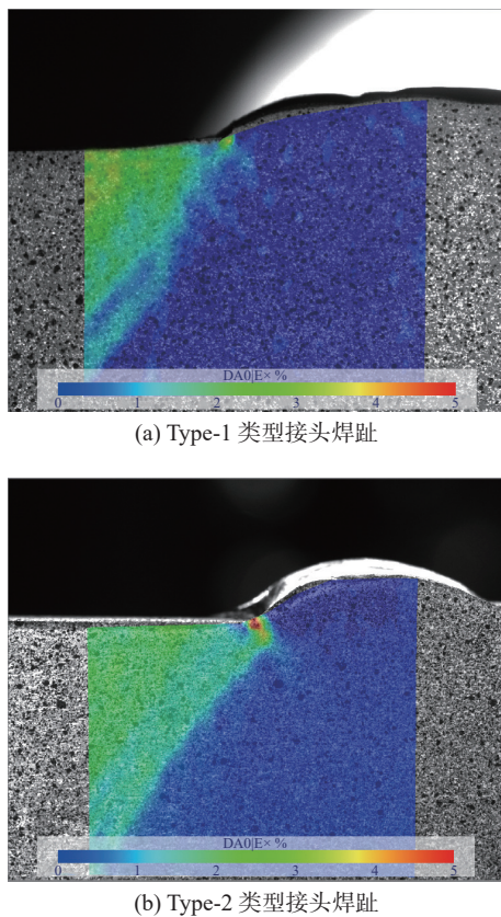
图 8 两种类型接头焊趾处应力集中
