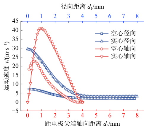
图 5 电极下方 2 mm 位置处径向和电弧中心轴向等离子体运动速度分布曲线
