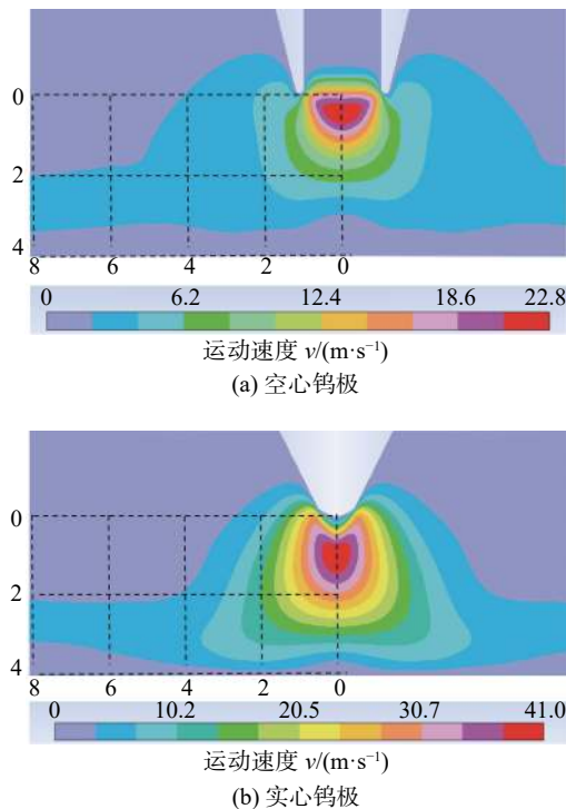
图 4 电弧等离子体运动速度分布云图 (mm)
