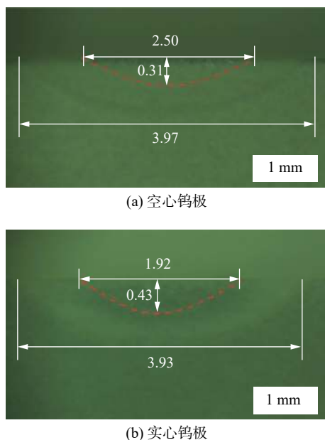
图 11 试验焊缝截面 (mm)
