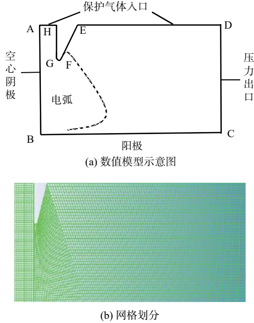
图 1 空心钨极 TIG 焊电弧数值模型及网格划分
