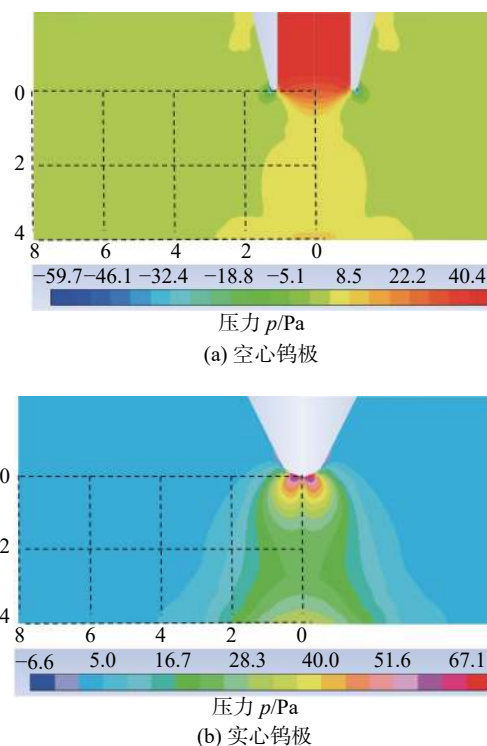
图 6 电弧压力分布云图 (mm)
